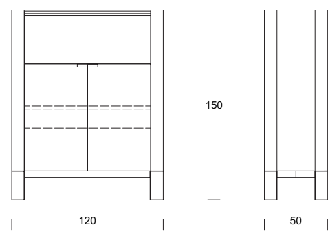
DUE ANTE CON CASSETTO + VANO GIORNO TWO DOORS WITH DRAWER + DAY COMPARTMENT
